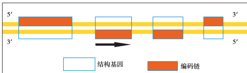
图 9-3 不对称转录
