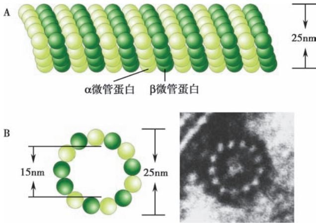
图 7-2 微管的结构
