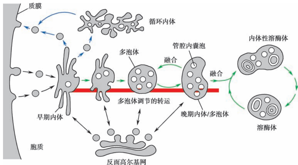
图 5-13 内体的成熟
