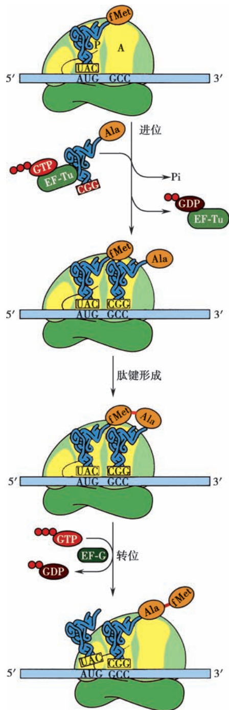
图 9-12 核糖体循环
