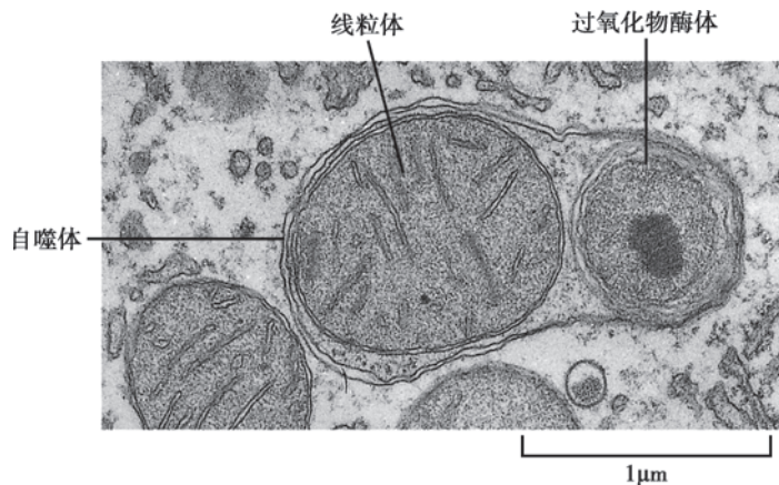
图 5-15 自噬体
