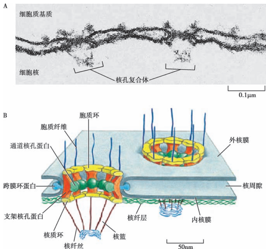
图 8-2 核膜的结构
