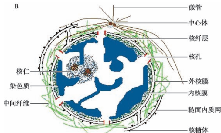
图 8-1 细胞核结构
